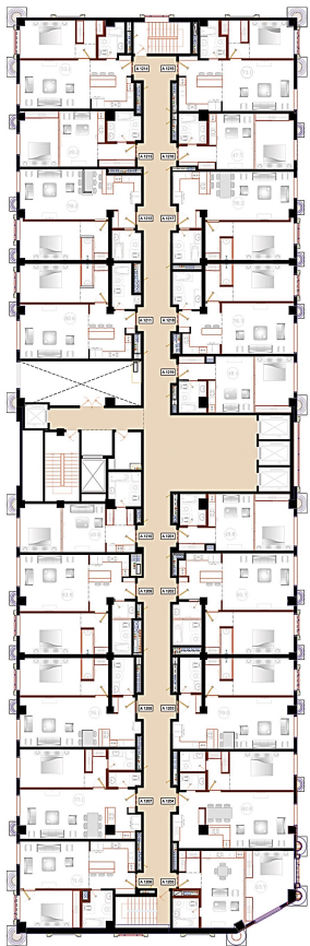
■ پلان طبقات FLOORS PLAN
